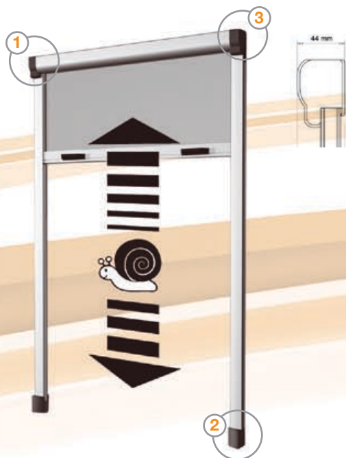
“ROTO” Zanzariera avvolgibile verticale Vertical roll-up insect screen
